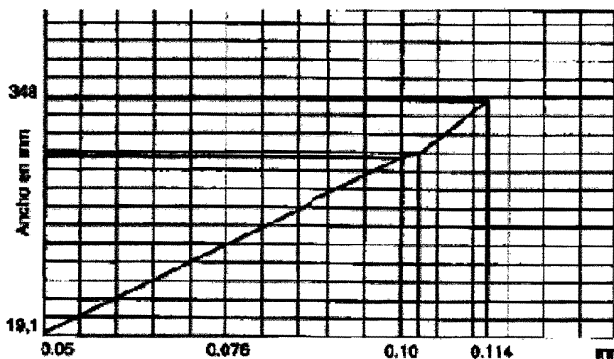
Gráfico de la relación entre el ancho y el huelgo de la unión.
