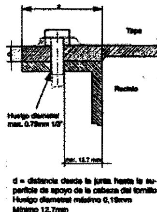
Ubicación del tornillo
