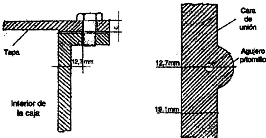
Posiciones de los agujeros en las uniones.
